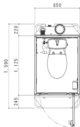
平面図 S=1/30
