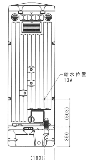
C 立面図 S=1/30
