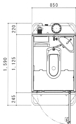
平面図 S=1/30
