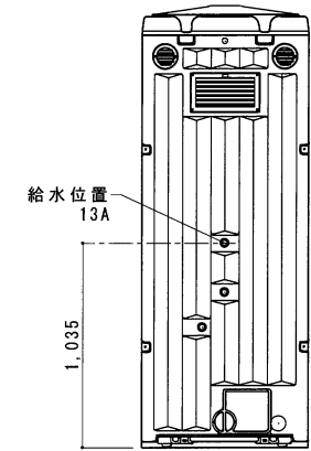
C 立面図 S=1/30
