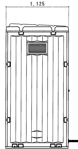
D 立面図 S=1/30
