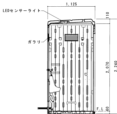
断面図 S=1/30
