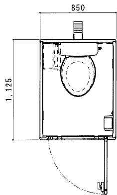
平面図 S=1/30
