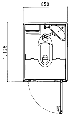
平面図 S=1/30
