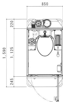
平面図 S=1/30
