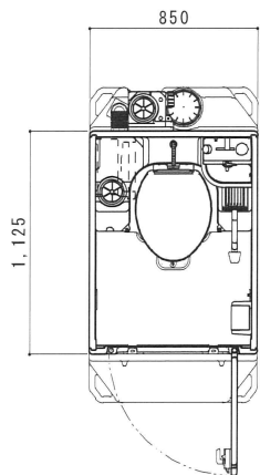
平面図 S=1/30
