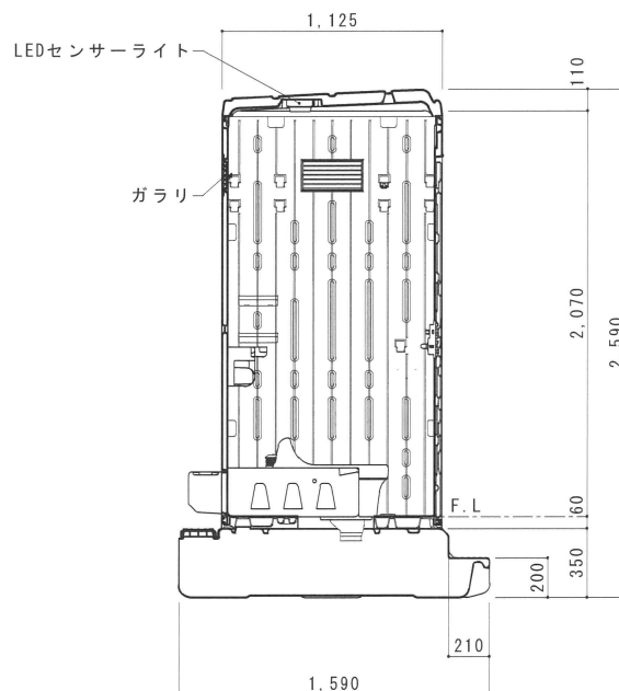
断面図 S=1/30
